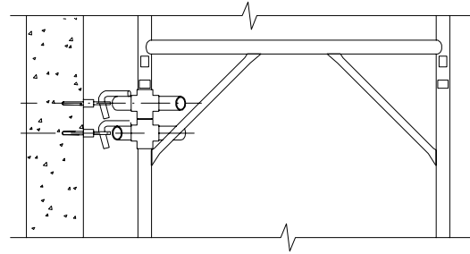
ANCORAGGIO A " V " CON STOCCO E TASSELLO MECCANICO / CHIMICO
