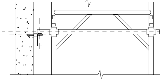
ANCORAGGIO " tipo A " CON TUBO Ø 48.3 x 3.2 E TASSELLO MECCANICO / CHIMICO
