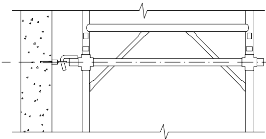
ANCORAGGIO CON STOCCO CON TONDINO E TASSELLO MECCANICO / CHIMICO
