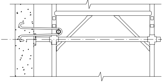
ANCORAGGIO AD ANELLO A TRAZIONE
