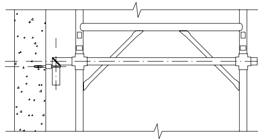
ANCORAGGIO " tipo B " CON TUBO Ø 48.3 x 3.2 E TASSELLO MECCANICO / CHIMICO
