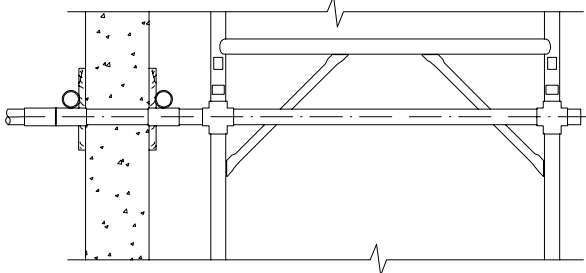
ANCORAGGIO A CRAVATTA
