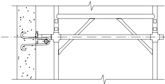
ANCORAGGIO AD ANELLO A SBADACCHIO
